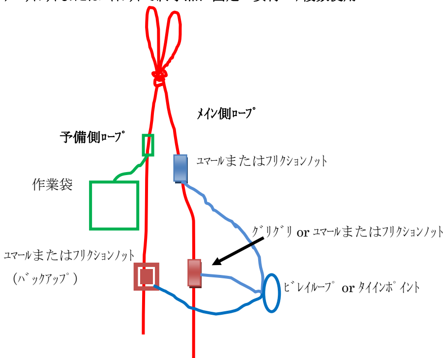
ビレー要領図
